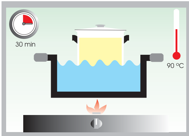
Fig. 5. Esterilização de 240 mL de leite ( 90^{\circ}\text{C} , durante 30 minutos).
