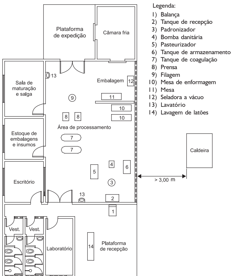
Fig. 32. Planta baixa da agroindústria de queijo prato.
