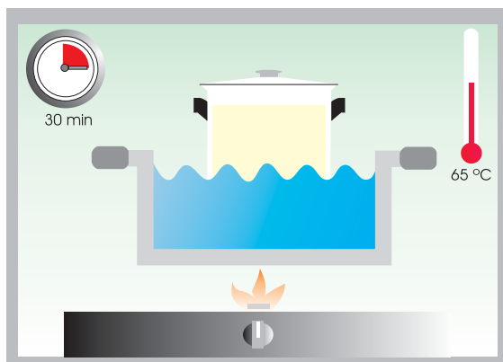
Fig. 2. Pasteurização do leite (65°C, durante 30 minutos).
