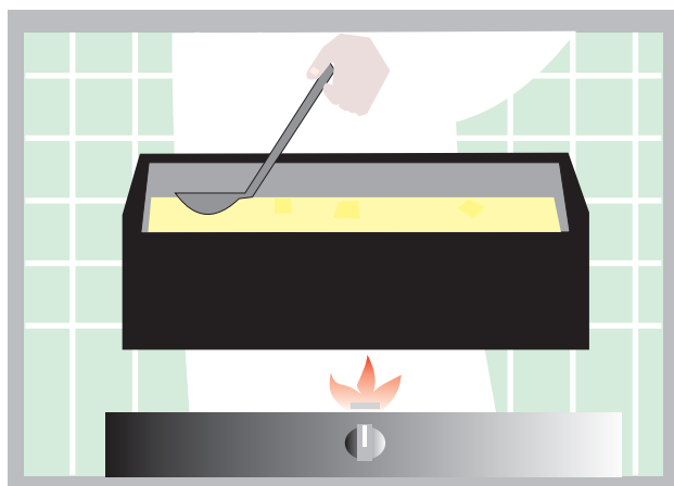
Fig. 22. Cozimento da massa (aumentar 1°C a cada 2 minutos).
