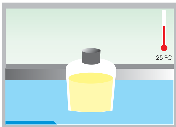
Fig. 6. Resfriamento do leite ( 25^{\circ}\text{C} ).
